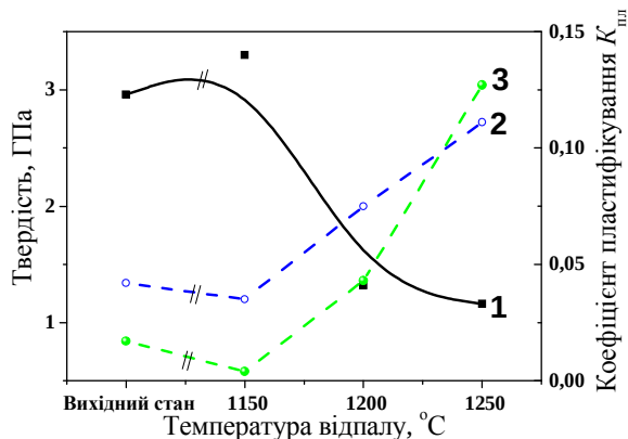
Рис. 8. Вплив температури відпалу на показники твердості HM та коефіцієнта пластифікування K_{пл} зразка ІМ Ni_3Al за умов інструментального (локального) індентування та статичного і динамічного навантажень: 1 — HM ; 2 — K_{пл}^c ; 3 — K_{пл}^d .
