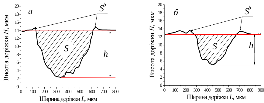
Рис. 4. Типові профілограми доріжок тертя інтерметаліду \text{Ni}_3\text{Al} в парі з індентором ШХ-15, отриманих при квазістатичному (а) та динамічному (б) режимах випробувань: h , S — глибина та площа доріжки тертя; S^b — площа витисненого матеріалу.
