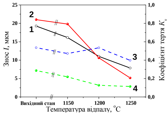
Рис. 7. Вплив температури відпалу на показники зносу I та коефіцієнта тертя K_T зразка ІМ Ni_3Al за умов статичного та динамічного навантажень: 1 — I^c ; 2 — I^d ; 3 — K_T^c ; 4 — K_T^d .
