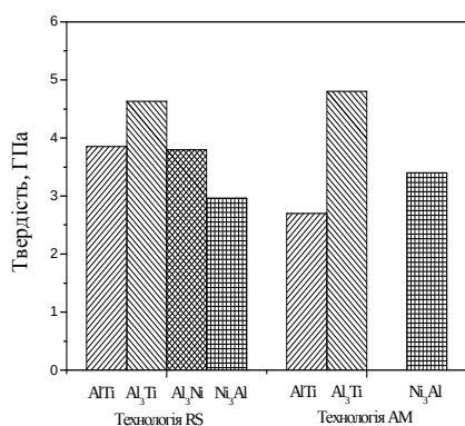
Рис. 6. Залежність твердості по Мейєру зразків ІМ AlTi, Al 3 Ti, Al 3 Ni, Ni 3 Al, виготовлених за різними технологіями.
