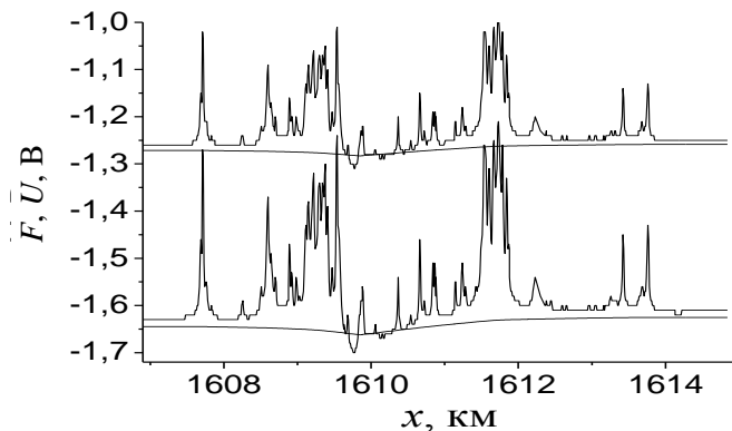
Рис. 4. Зміна потенціалів F, U_c вздовж трубопроводу за умови величини струму 12,9 А (нижні графіки) і 8,5 А (верхні графіки).
