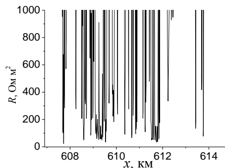
Рис. 3. Зміна опору R на окремих ділянках трубопроводу.
