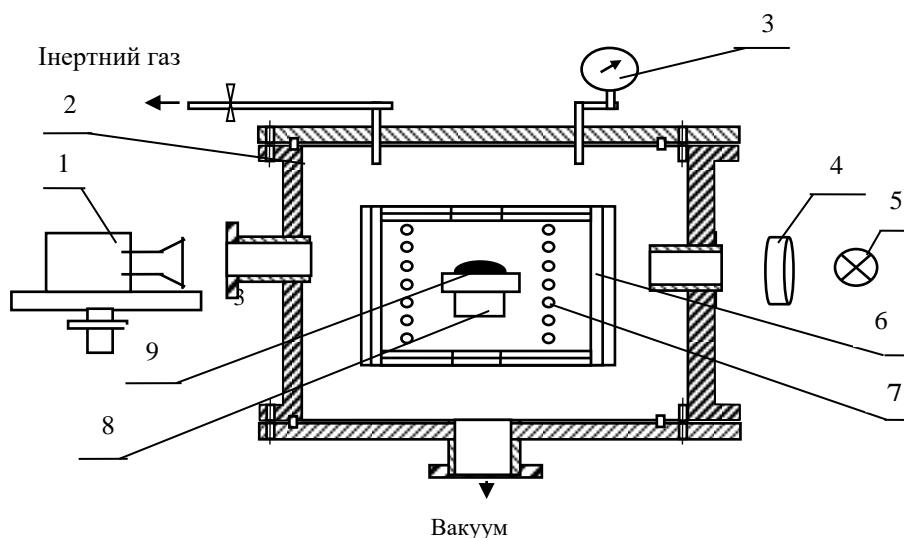
Рис. 1. Схема вакуумної установки для плавлення/синтезу металів: 1 — фото- або відеокамера; 2 — вакуумна камера; 3 — манометр; 4 — конденсор; 5 — освітлювальна лампа; 6 — екран; 7 — нагрівач; 8 — столик; 9 — підкладка (тигель) з краплею металу [8].
