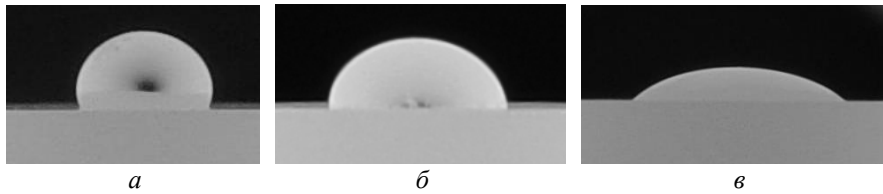
Рис. 6. Рідкі краплі металів на поверхні діоксиду олова: a — срібло (1273 К); б — мідь (1373 К); в — олово (1073 К).
