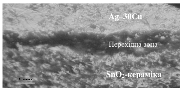
Рис. 11. Мікроструктура зони контакту SnO 2 -кераміка/Ag—30Cu розплав.
