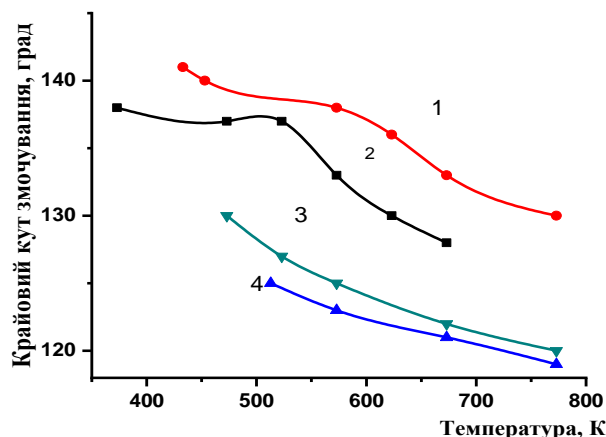
Рис. 2. Температурна залежність крайового кута змочування \text{In}_2\text{O}_3 розплавленими металами та сплавами у вакуумі: 1 — індій; 2 — галій; 3 — ПОС-61; 4 — олово.
