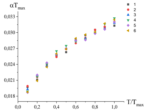
Рис. 1. Залежність \alpha \cdot T_{\max} від гомологічної температури для матеріалів Ni (1), NiCoCr (2), MiCoCrFe (3), Fe (4), TiZrVNBa (5), WNBMoTaV (6).
