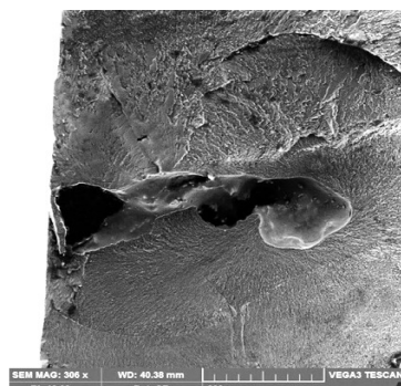
Рис. 8. Пори в зоні наплавленого металу зразків № 1 ( a ) та 2 ( б ).
