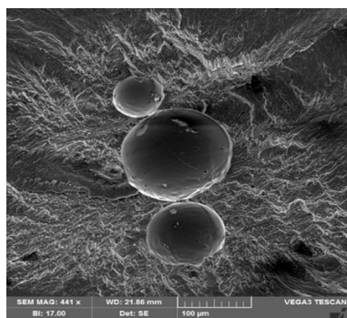
Рис. 8. Пори в зоні наплавленого металу зразків № 1 ( a ) та 2 ( б ).
