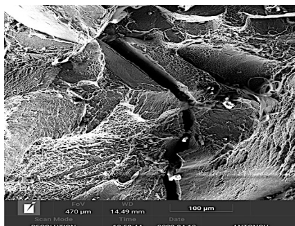
Рис. 9. Фотографії втомного мікрорельєфу в зоні наплавлення зразків № 1 ( a ) та 2 ( б ).
