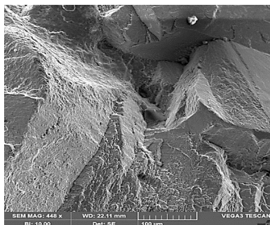
Рис. 9. Фотографії втомного мікрорельєфу в зоні наплавлення зразків № 1 ( a ) та 2 ( б ).
