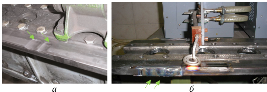
Рис. 1. Фотографія ділянки, де відбувся знос робочої поверхні рейки літака Ан-124, (а) та вид дефектної поверхні після застосування відновлювального наплавлення (б).
