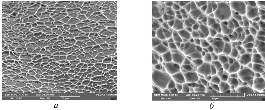
Рис. 11. В'язкий мікрорельєф у зоні долому зразків № 1 (а) та 3 (б).
